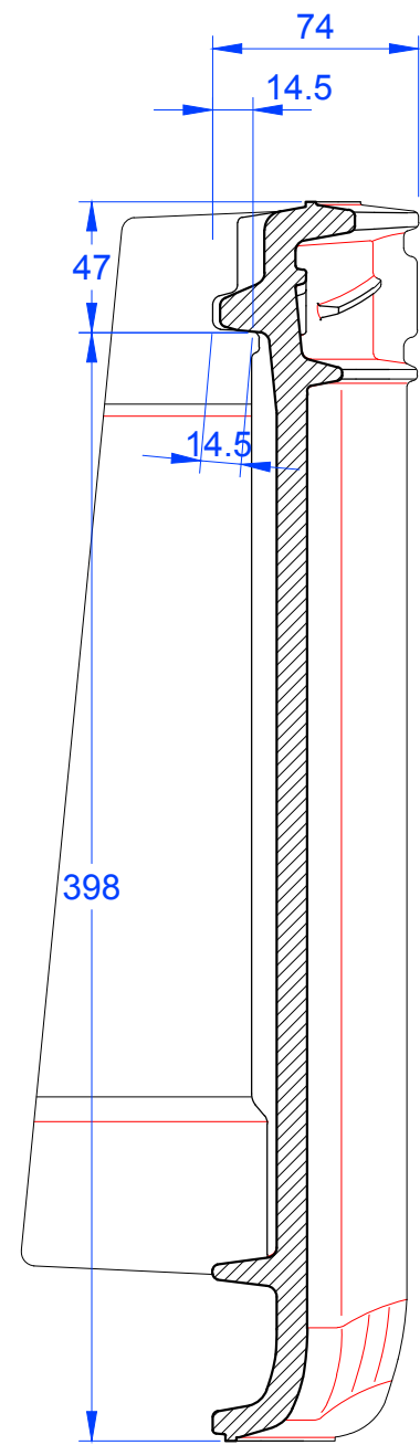
Schnitt B-B
