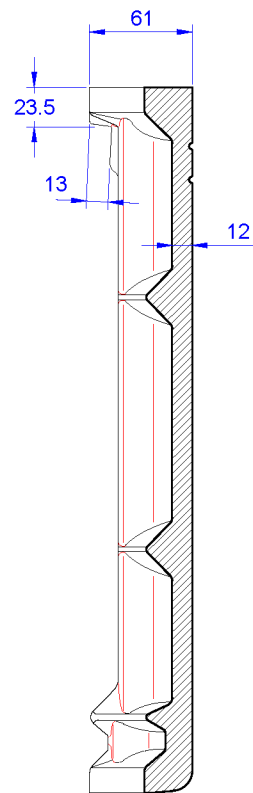
Schnitt B-B
