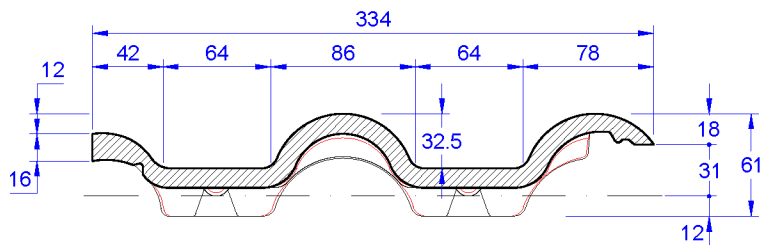
Schnitt A-A
