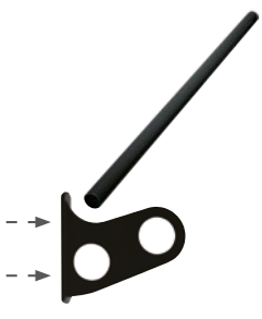
Wspornik do rur śniegowych Rura śniegowa Ø 40 Funkcja: 4080/4090
