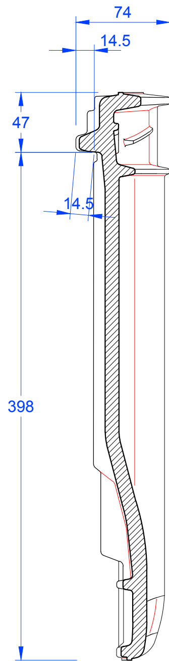
Schnitt B-B
