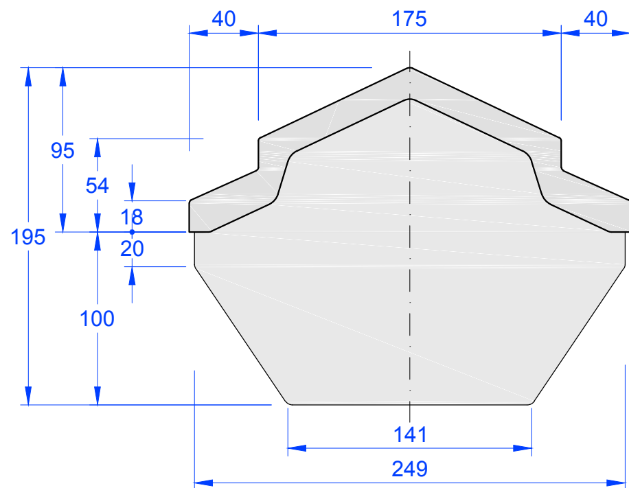
Ansicht von vorne
