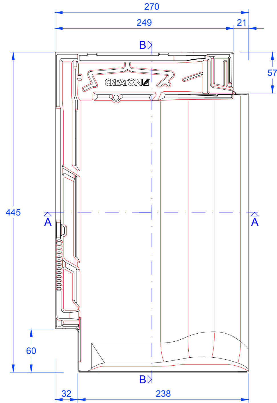
Schnitt A-A
